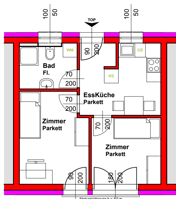
Variante B: ca. 36 m 2 2 Schlafzimmer
